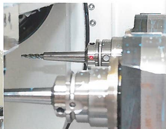
Das additiv gefertigte Hydrodehnspannfutter überzeuget nicht nur mit seiner schlanken Form.
